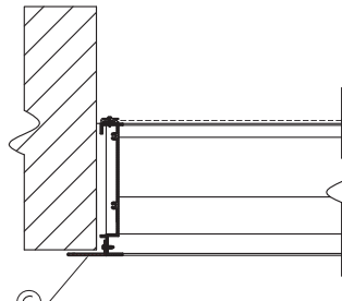
FLANGE FRAME
